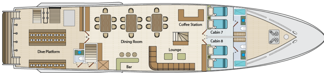
LOWERDECK
